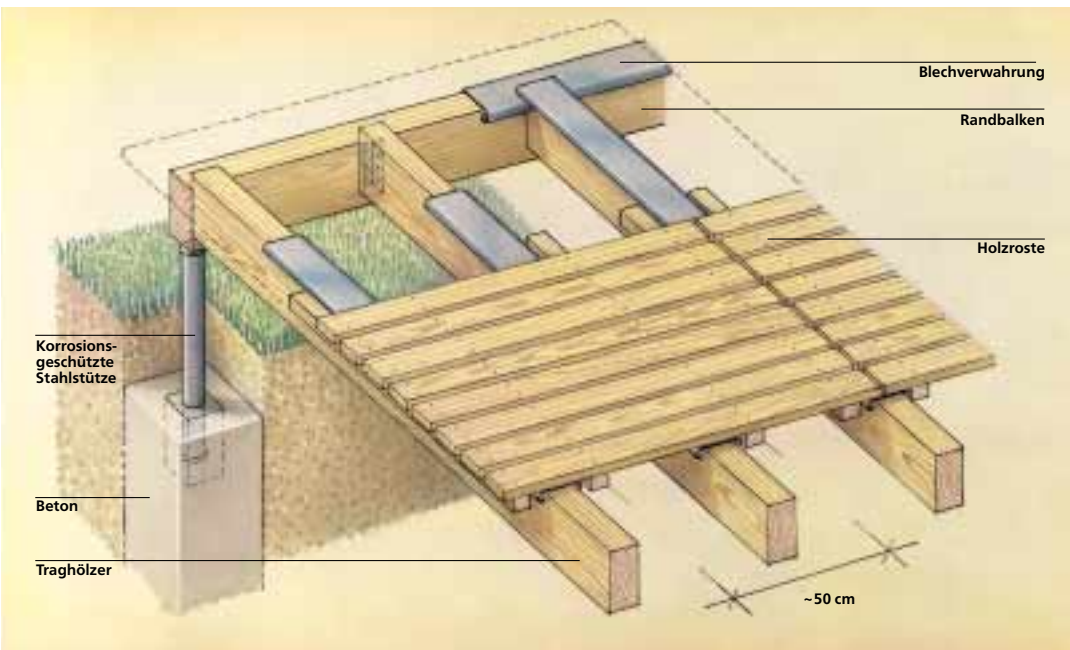
Abb. 32: Beispiel aufgeständerte Terrasse
